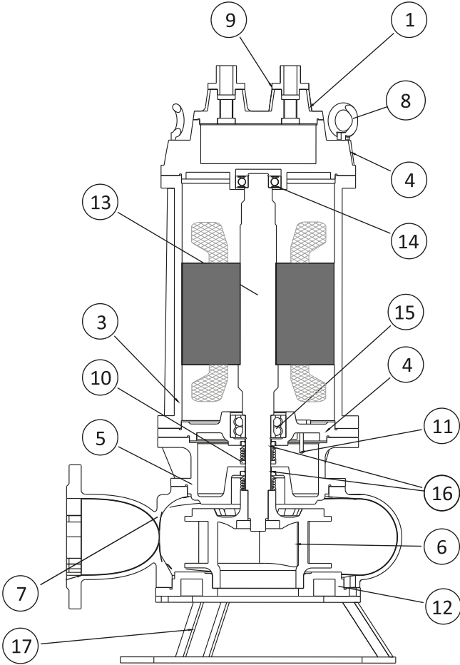
Kesit Resmi / Sectional Drawing
